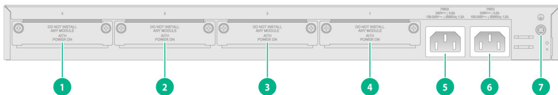
图1-2 R3900-S28-G-DP 后视图
