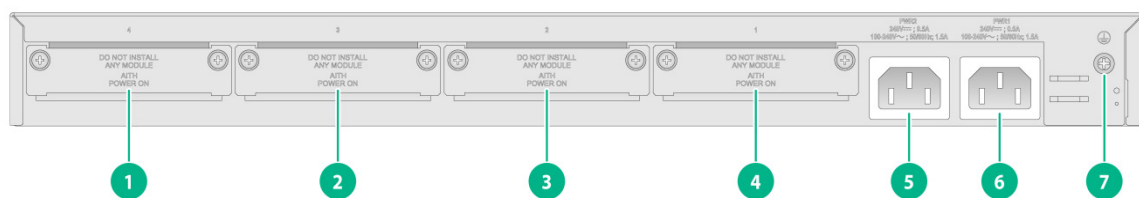
图1-4 R3900-S51-G-DP 后视图
